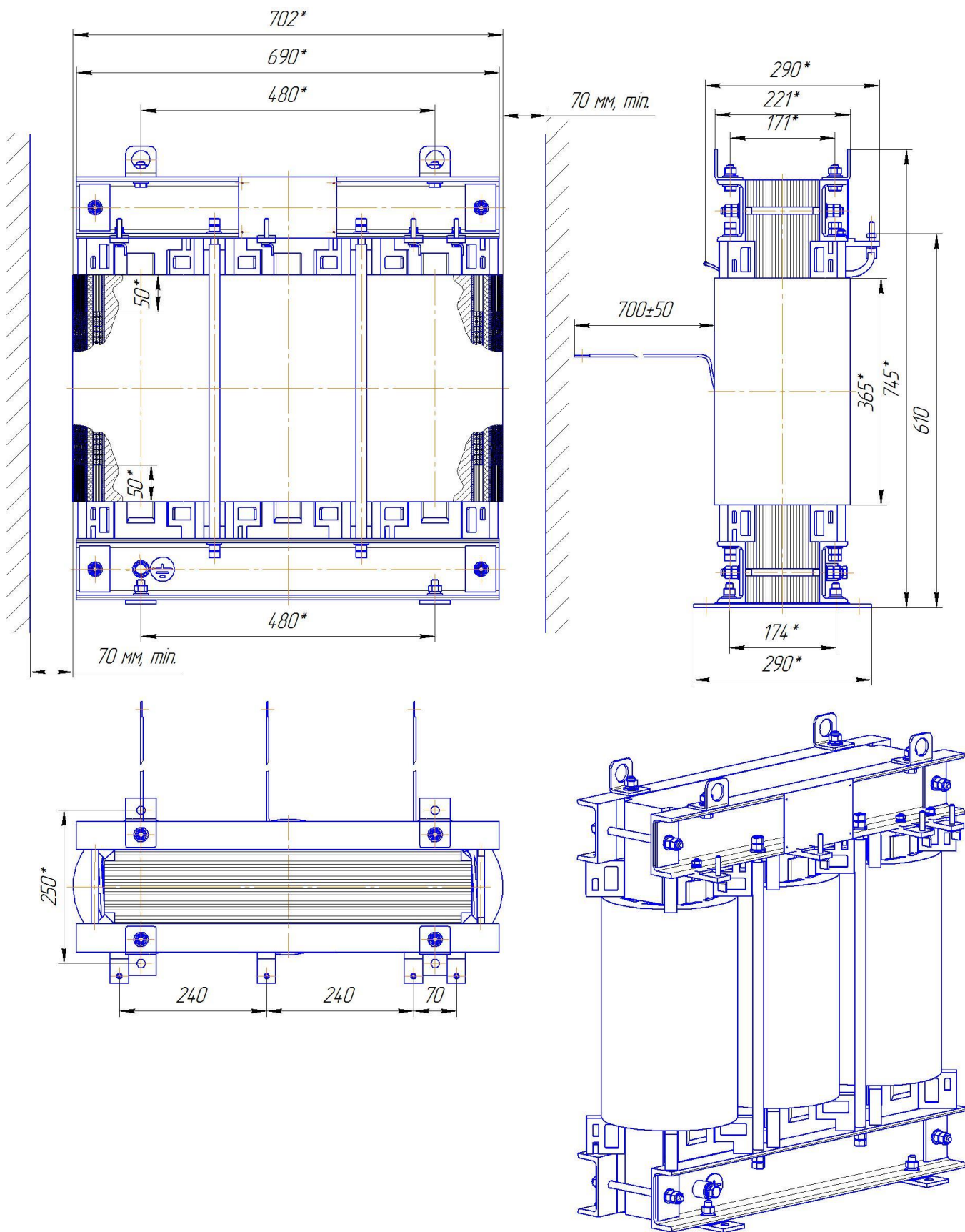
Рисунок 1 - Общий вид, габаритные, установочные и присоединительные размеры трансформатора типа ТСКС-40/145/6 – УЗ.
